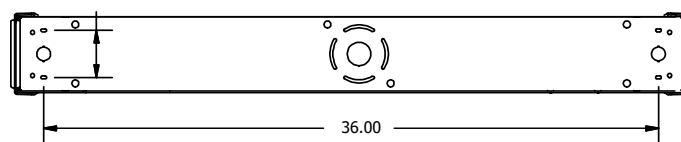
3' Dimensions finales
